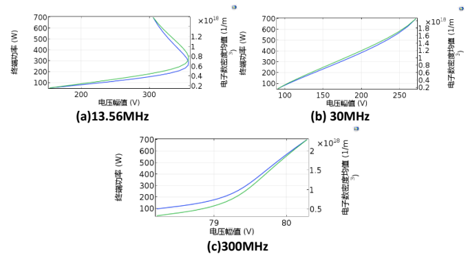
图 6 不同频率下的放电特性曲线
