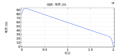
(c)300MHz, 627W
