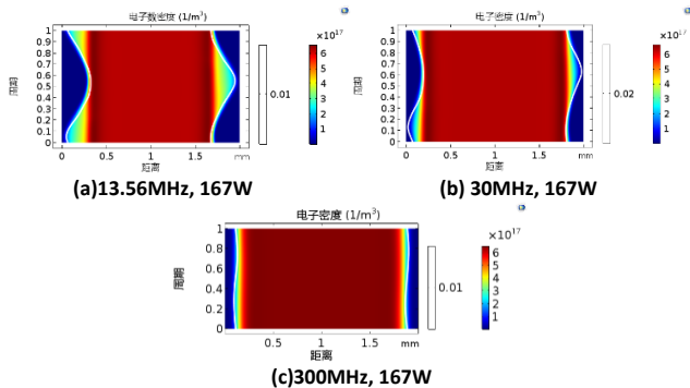
图 3 不同频率下的鞘层厚度
