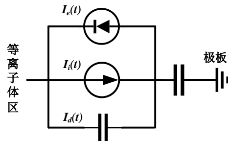
图 2 射频等离子体鞘层等效电路模型
