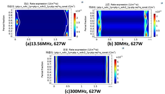
图 5 不同频率下的电离速率
